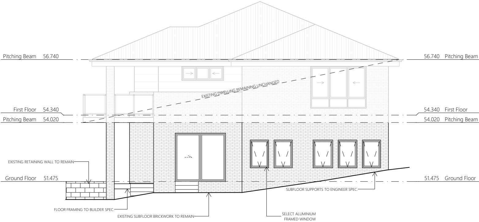
E02 Elevation 1:100
